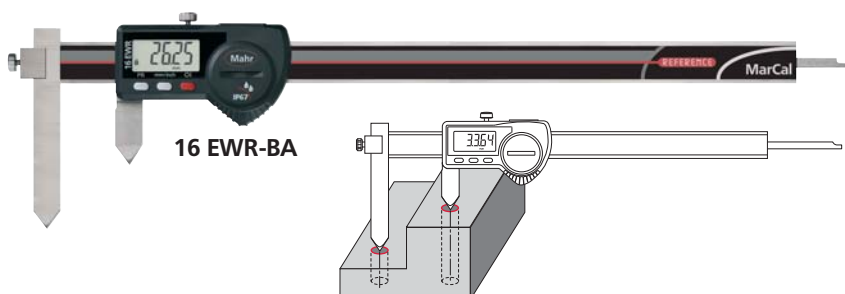
Pos. měřítko s posuvnou čelistí pro měření roztečí otvorů
