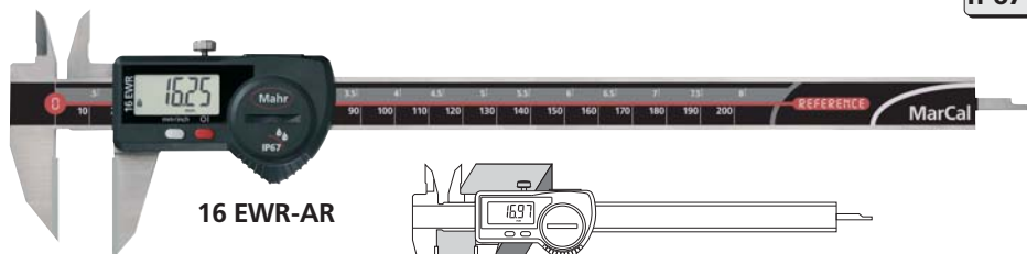
Pos. měřítko pro hřídel. drážky
